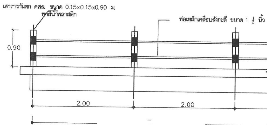
แบบขยายราวกันตก มาตราส่วน
