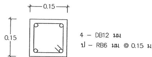
แบบขยายเสาขี้นวุ่นตัวไฉ่ มาตราส่วน
