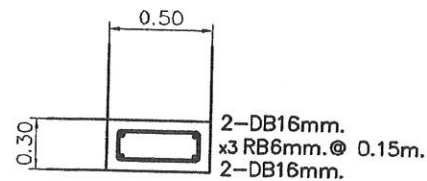
แบบขยายคานทับหลัง
