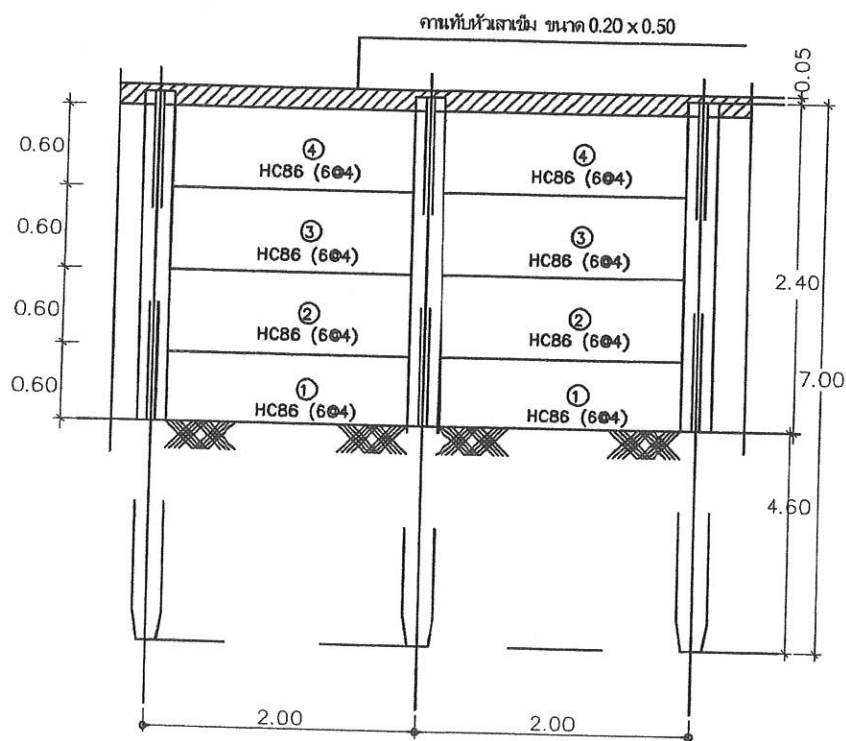
รูปด้านผนังกันดิน
