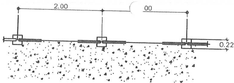
แบบแปลนผนังกันดิน
