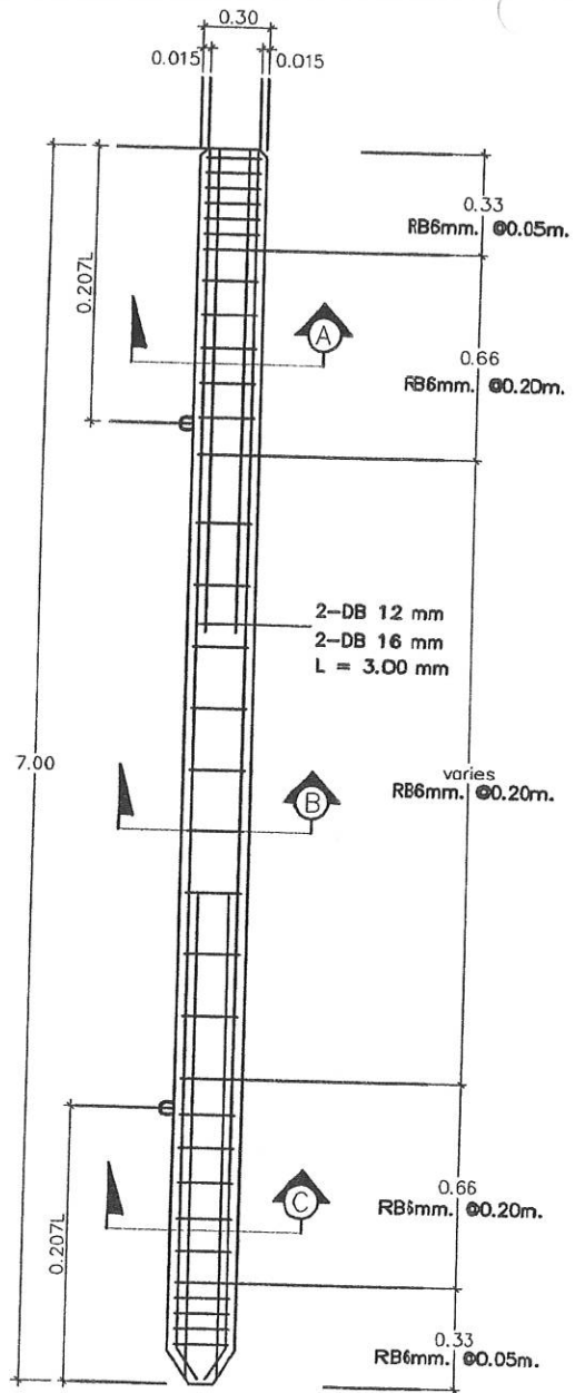
แบบแสดงการเสริมเหล็ก
